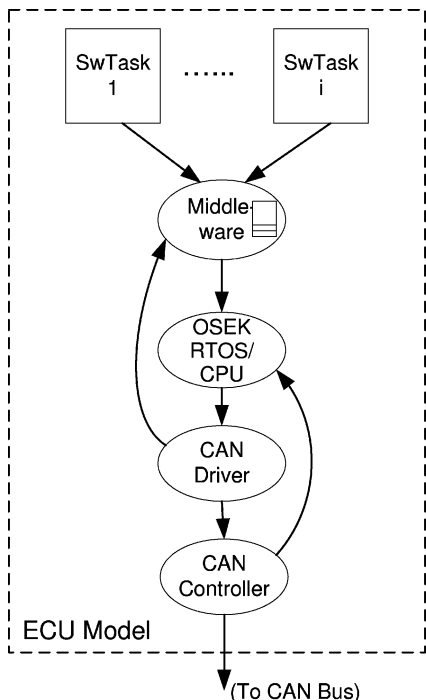
Fig. 13. ECU model.
